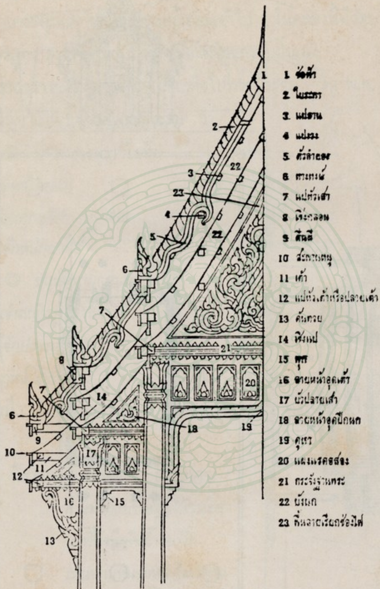
ภาพลายเส้นแสดงข้อส่วนของอาคาร ตามแบบ สถาปัตยกรรมไทย เปรียบเทียบกับพระอุโบสถวัดปราสาท
