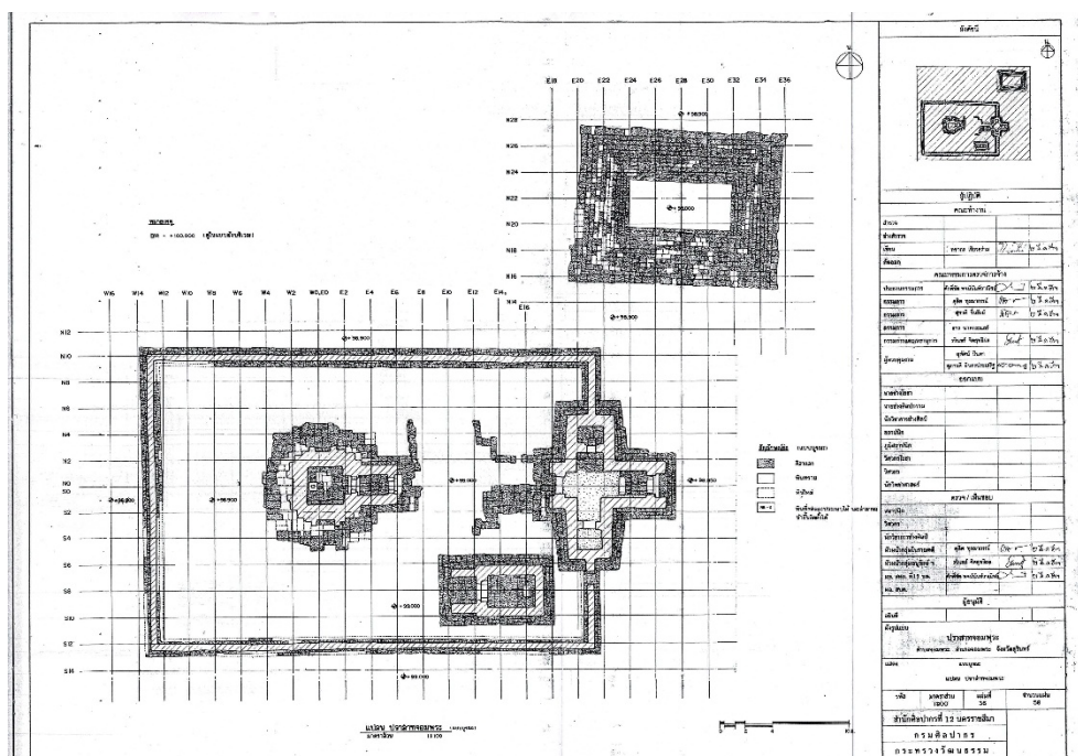
ภาพที่ ๒.๒ ผังบริเวณแสดงองค์ประกอบทางสถาปัตยกรรมของปราสาทจอมพระ
