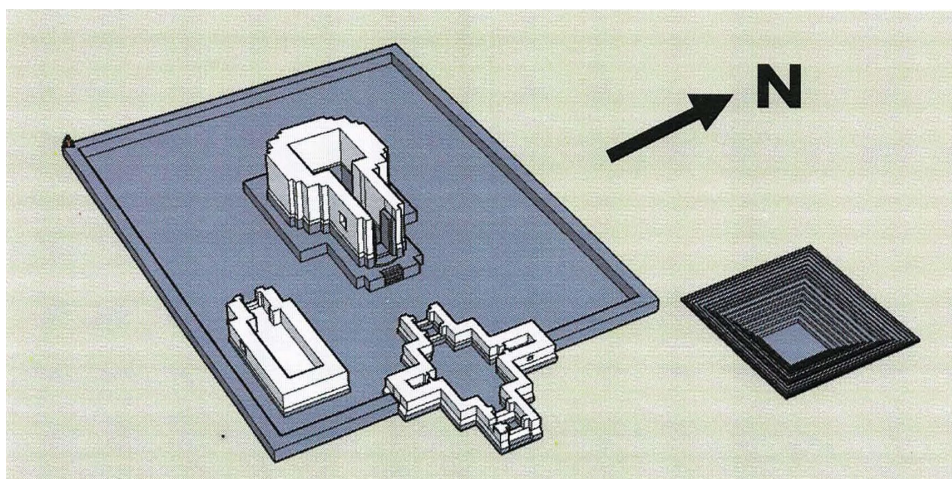
ภาพที่ ๒.๑ แผนผังโบราณสถานปราสาทจอมพระ
